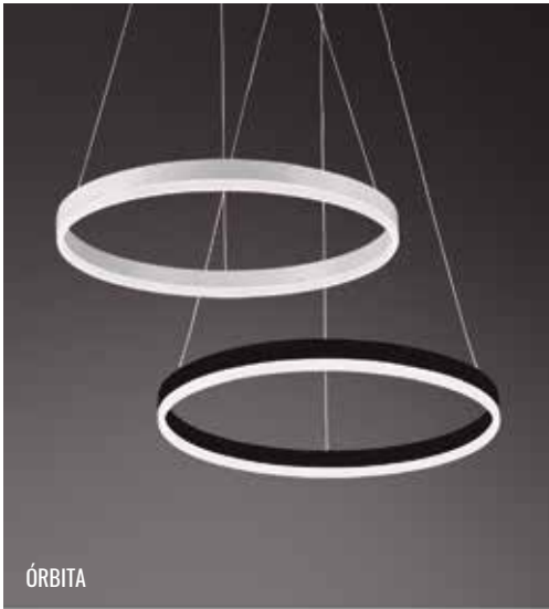
ÓRBITA Ø:600 mm | Alturas regulables hasta 1200 mm Material Metal + Acrílico 30W 3000K 1890 Lm ○ cód. 146929 ● cód. 146930
