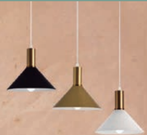
Ø:250 H:250 mm | Altura regulable hasta 1200 mm Material Aluminio + Metal 1xE27 MÁX 40W | No incluye foco cód. 146513 1xE27 MÁX 40W | No incluye foco cód. 146512 1xE27 MÁX 40W | No incluye foco cód. 146511
